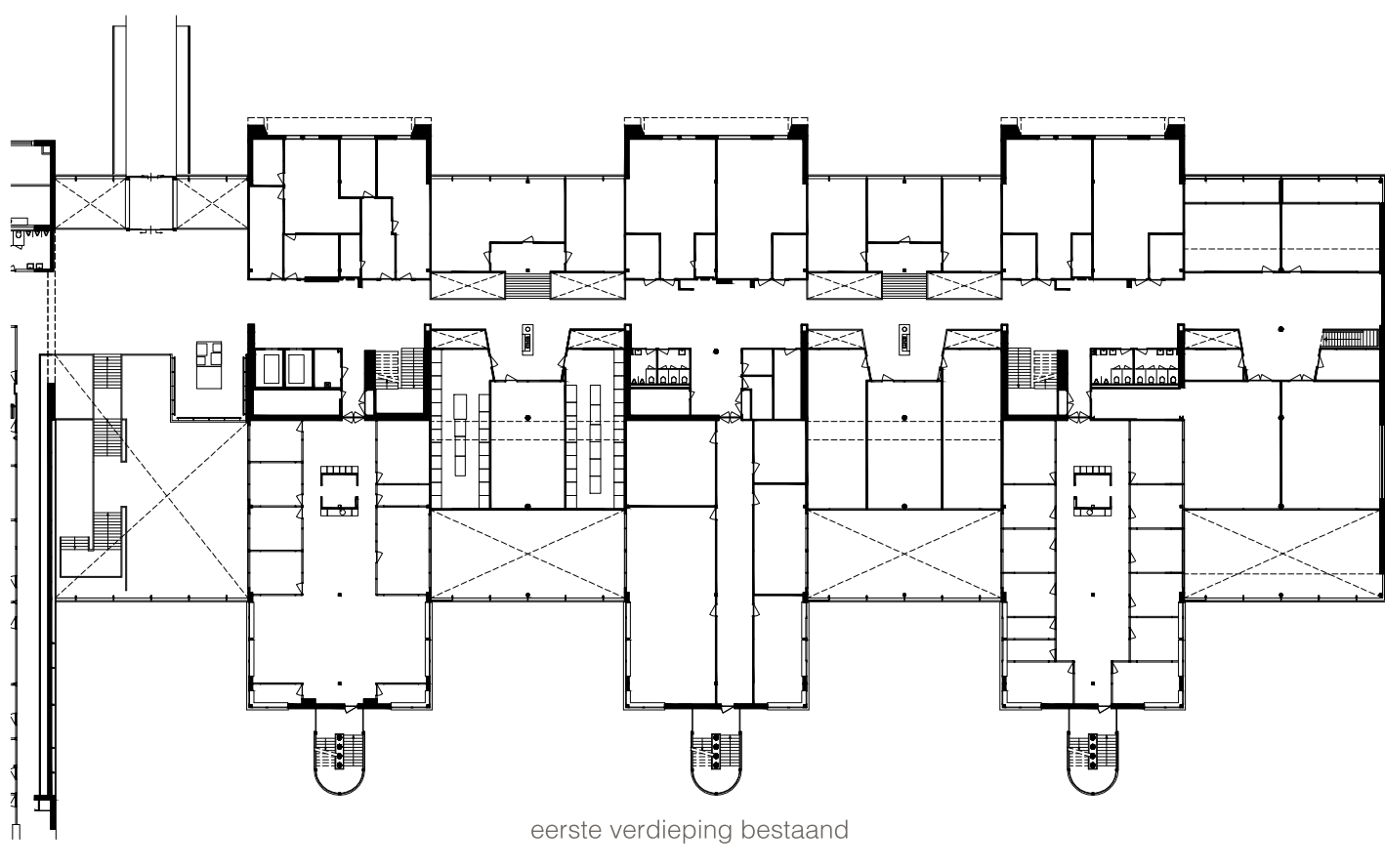
eerste verdieping bestaand
