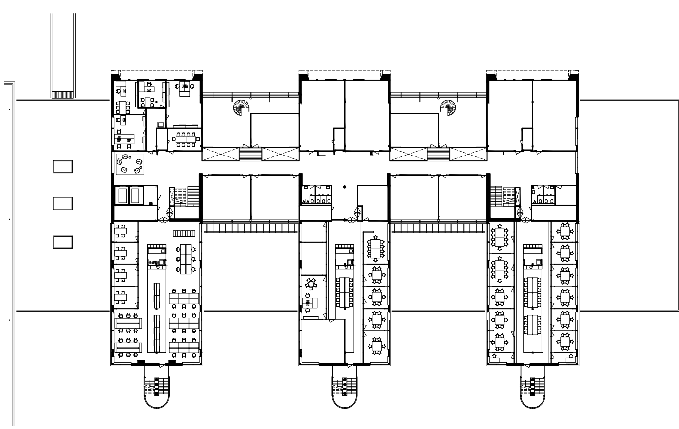
tweede verdieping nieuw
